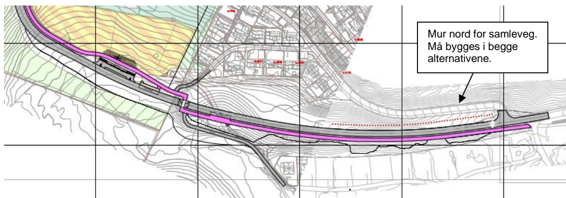
Figur 0-2 Forslag til alternativ løsning for gang- og sykkelveg med kryssing i plan.
