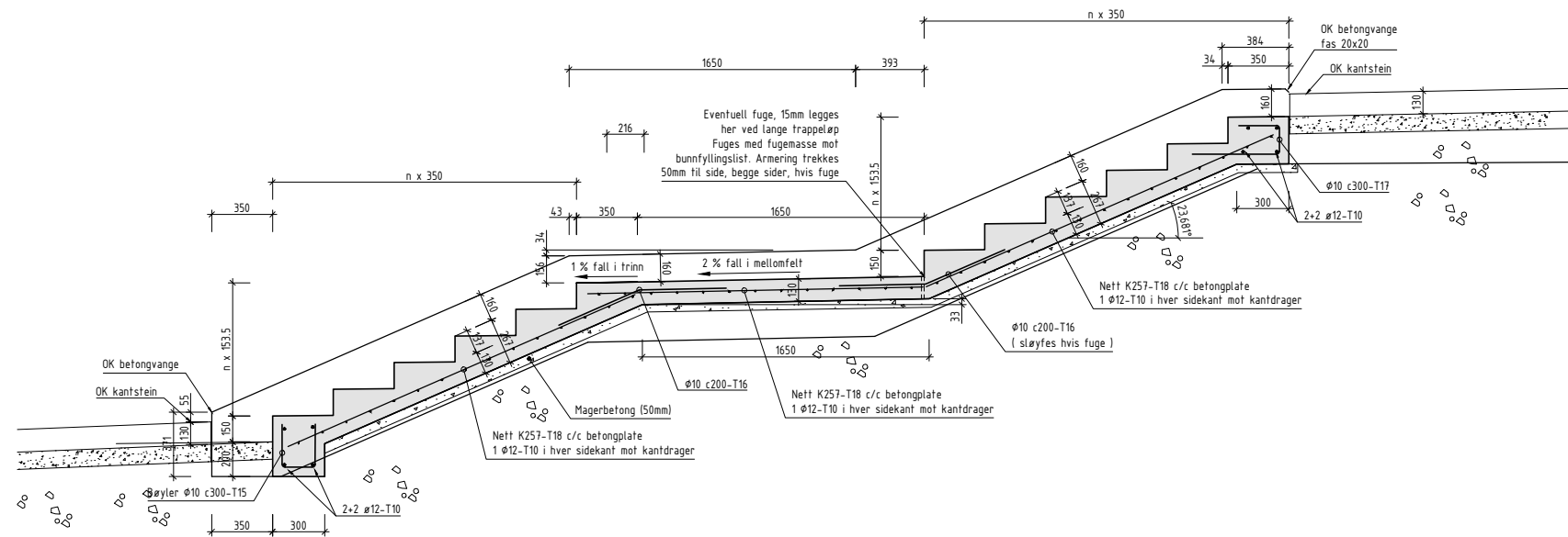
Oppriss trapp. (1:20) Prinsipp
