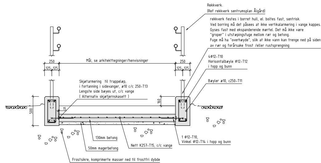
Tverrsnitt trapp. (1:20) Prinsipp
