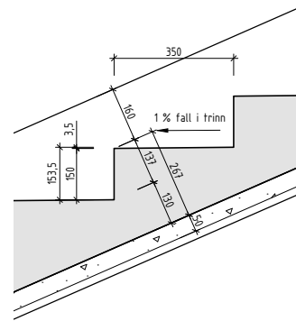
Detalj trinn (1:10)
