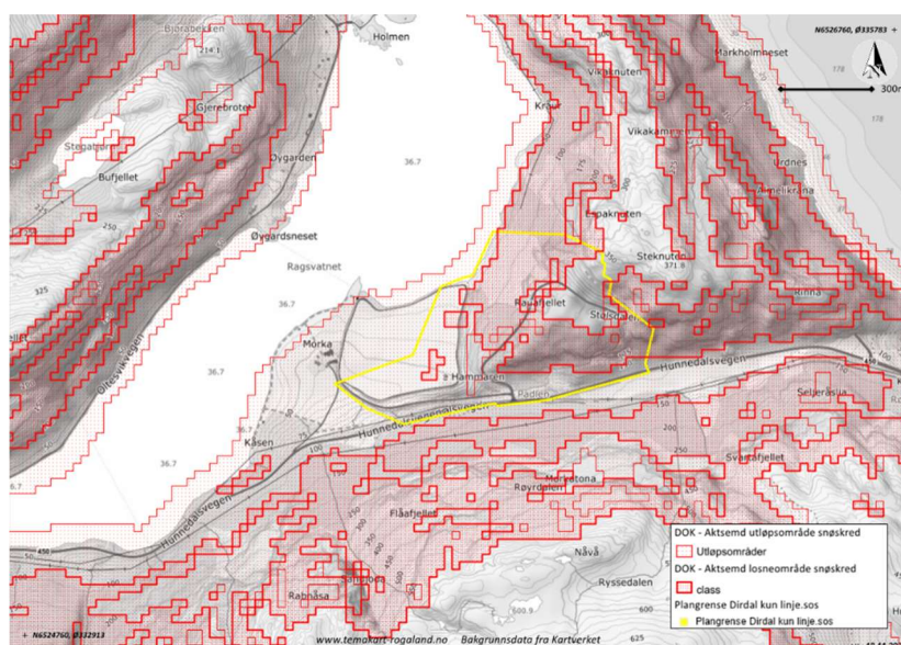
Figur 13 Aktsomhetsområder for snøskred. Kilde: temakart-rogaland.no
