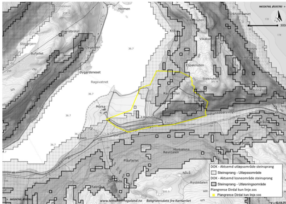
Figur 14 Aktsomhetsområder for steinsprang. Kilde: temakart-rogaland.no
