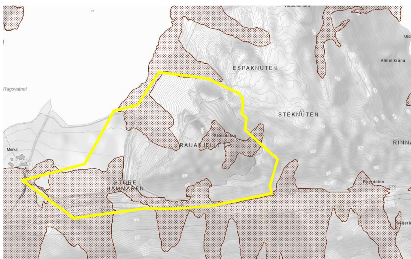
Figur 12 Aktsomhetsområde jord- og flomskred. Kilde: NVE
