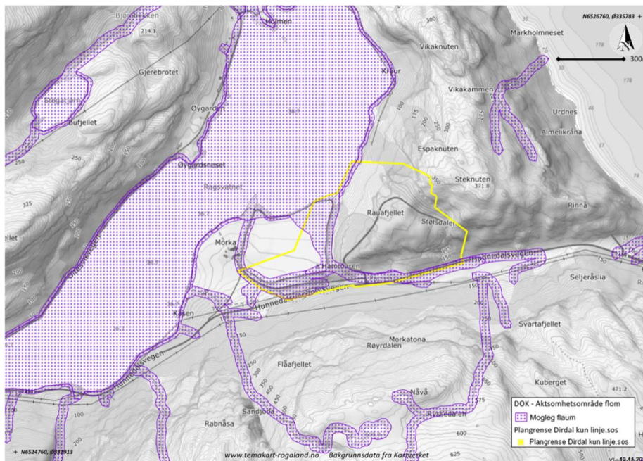
Figur 15 Aktsomhetsområde flom. Kilde: temakart-rogaland.no
