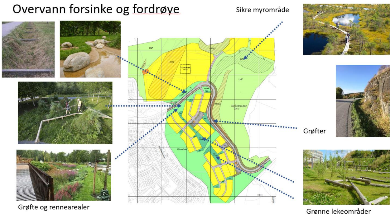
Figur 23 Prinsipper for å forsinke og fordrøye.
