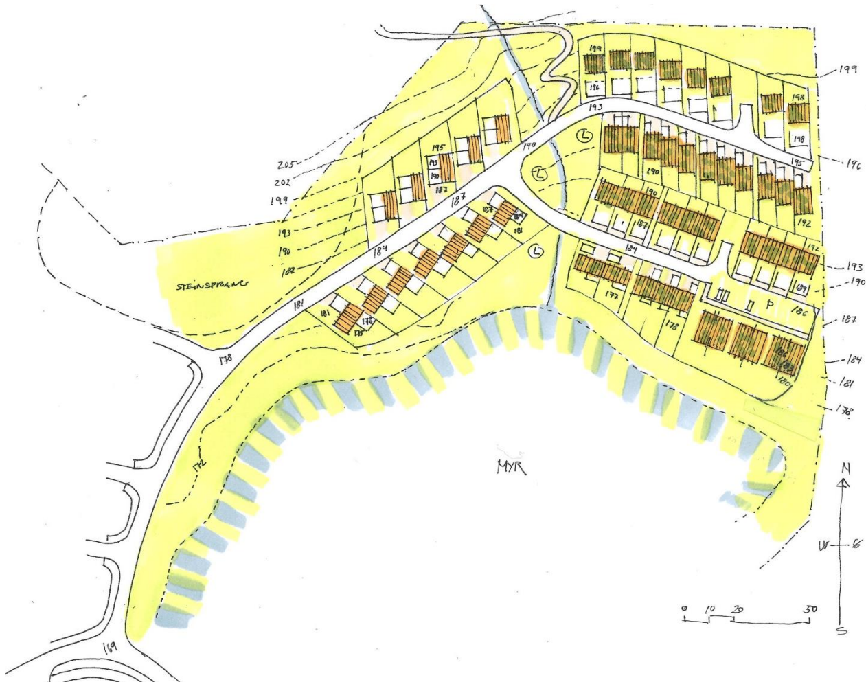
Figur 21 Illustrasjonsskisse for utvikling av delområde D3.
