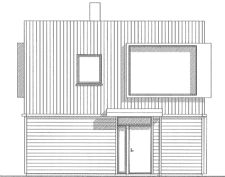
FASADE MOT VEST
