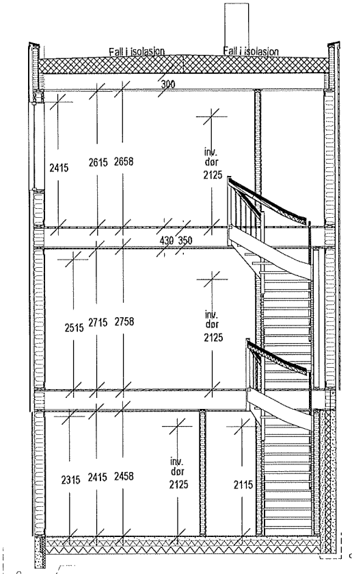
SNITT A-A
