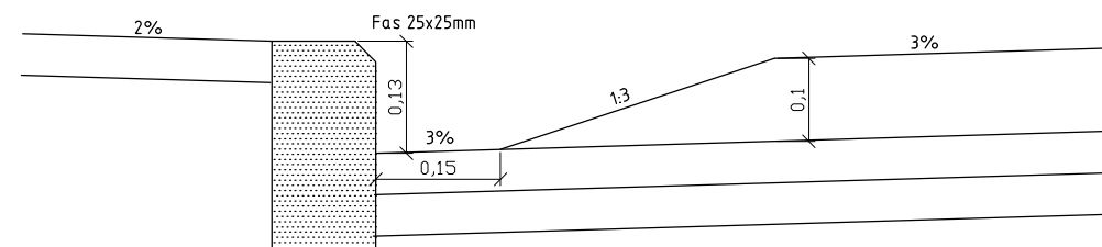
Detalj B, M=1:5 Tverrsnitt mot kantstein
